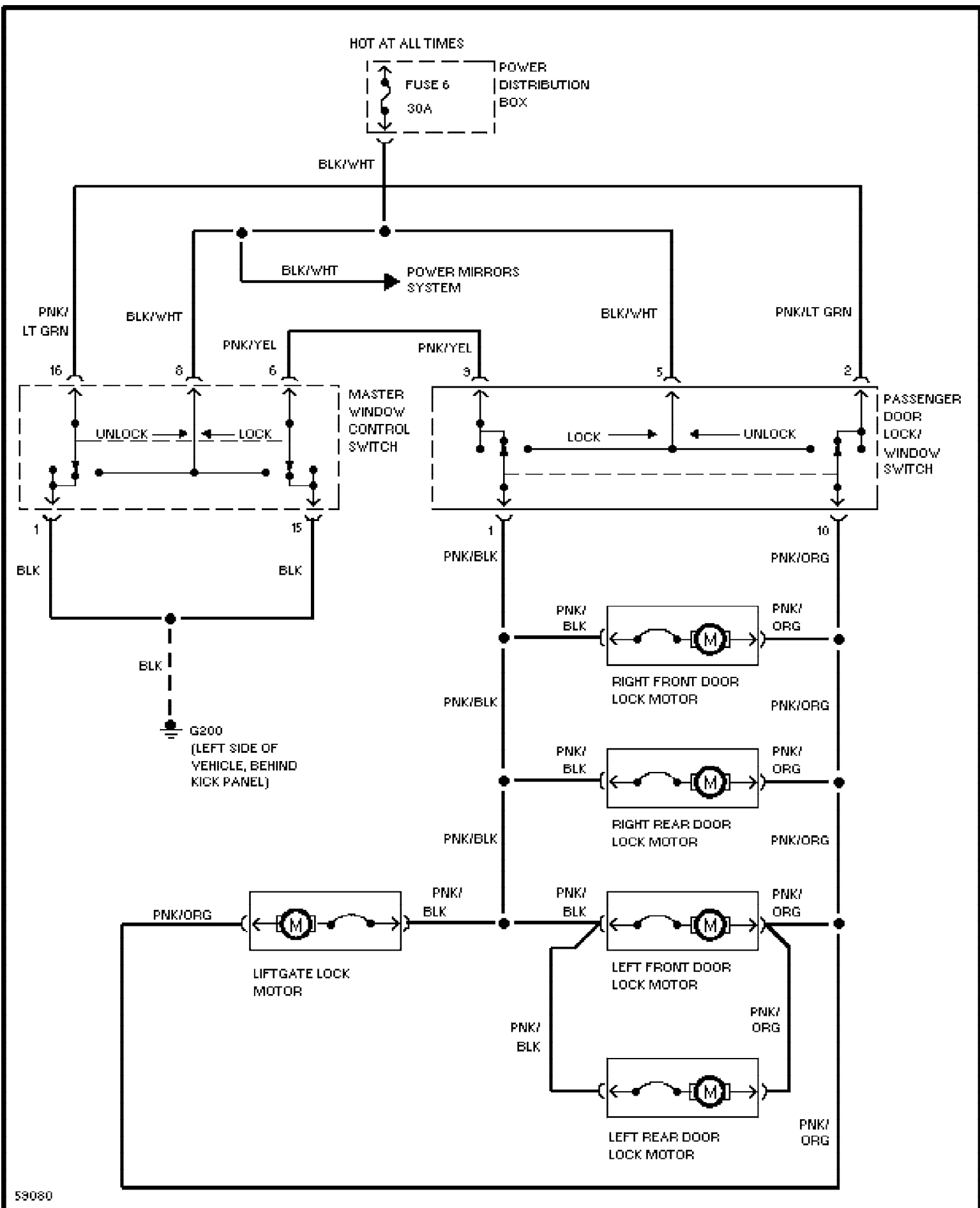
Fig. 30: Door Lock Circuit, 4 Door 1994 Ford Explorer
